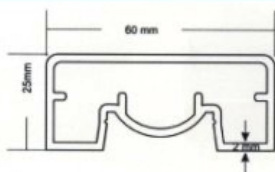
BRIDGE NT 2540 Madlo hranate 60x25 mm s oblukovov dražkov
