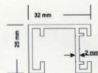
BRIDGE NT 2545 Profil na sklo 32 x 25 mm
