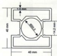
BRIDGE NT 2440 Stĺpik hranatý s dvomi dražkami
