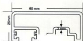
BRIDGE NT 2543 Madlo hranate 60x25 mm s dvomi dražkami
